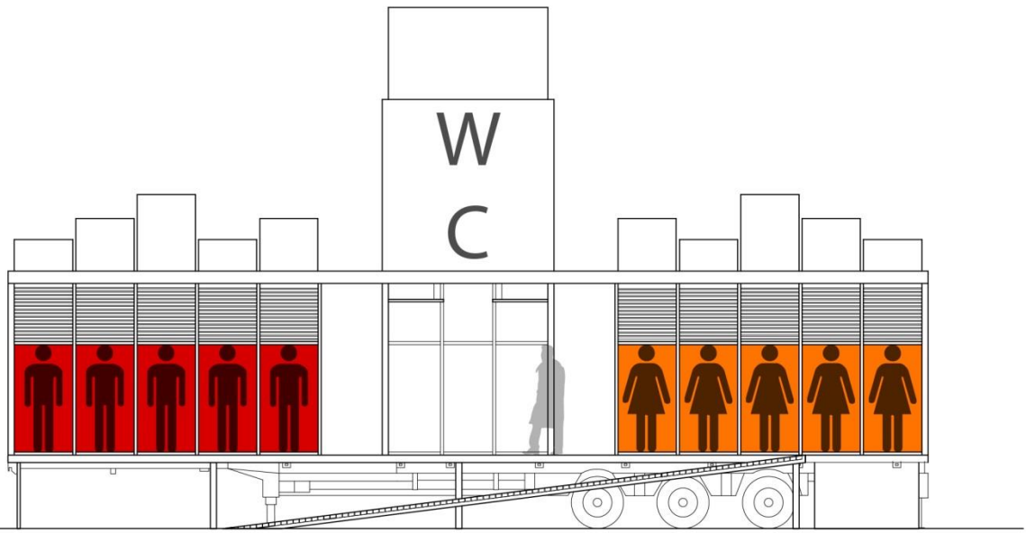
Elevation 1cm:1m
