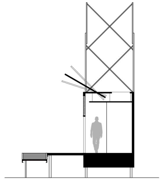
Section 1cm:1m
